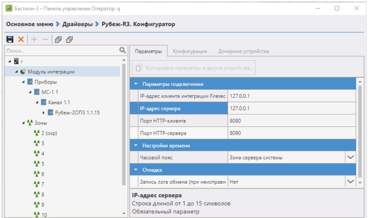
Рис. 3: Главное окно конфигуратора драйвера «Бастион-3 – Рубеж Прот. R3»
